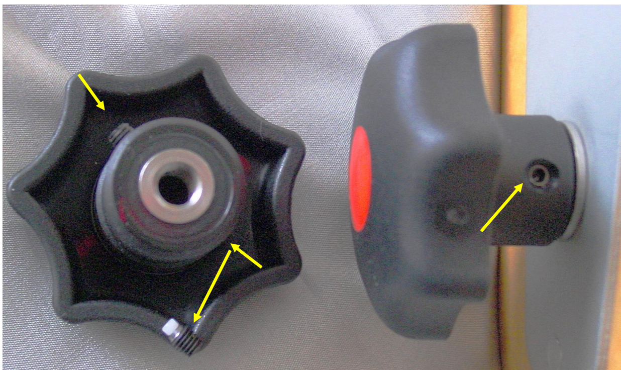
Drehgriff M 8 Ø gesamt L. ca. 38 mm
